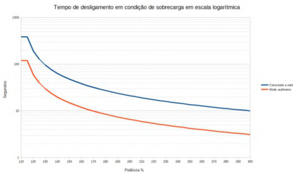
Gráfico do tempo suportado em condição de sobrecarga até ocorrer o desligamento da Saída AUX.
