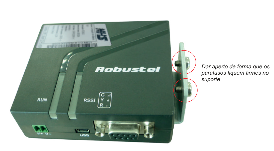
Figura 07: GPRS fixado e pronto para ser embalado
