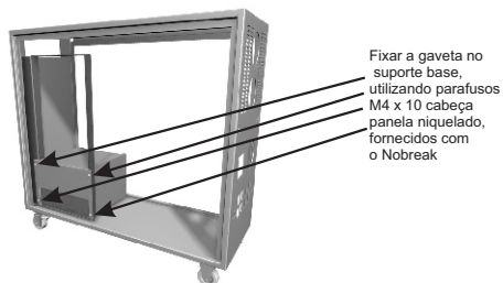
Fixação da primeira gaveta
