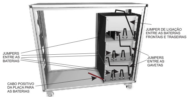
Fixação dos Jumpers ( Vista Lateral B )
