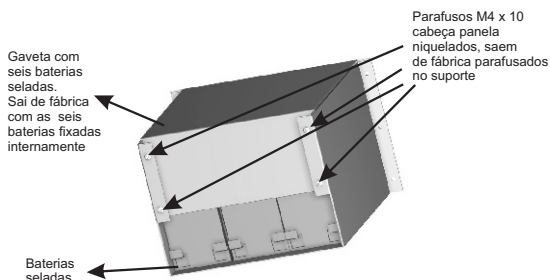
Gaveta com baterias seladas
