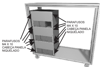
Fixação das gavetas restantes
