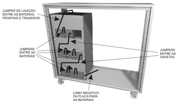
Fixação dos Jumpers ( Vista Lateral A )
